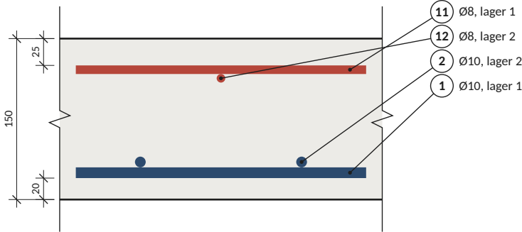
DETALJ F Armeringens lägen
