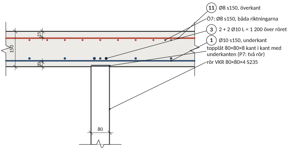
SEKTION B-B Vid rör (P5)
