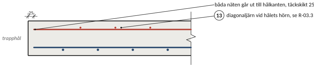
SEKTION C-C Trapphållets kant
